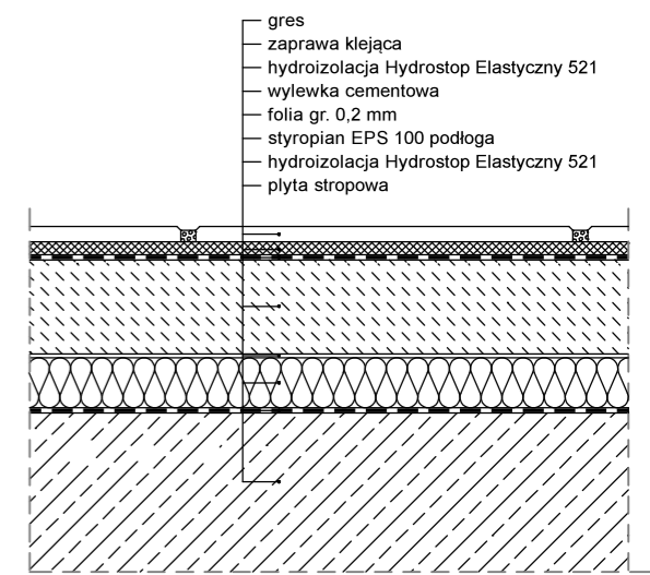
Przekrój przez warstwy podłogi
