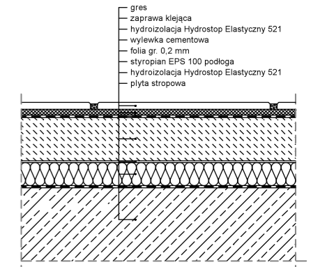
Przekrój przez warstwy podłogi
